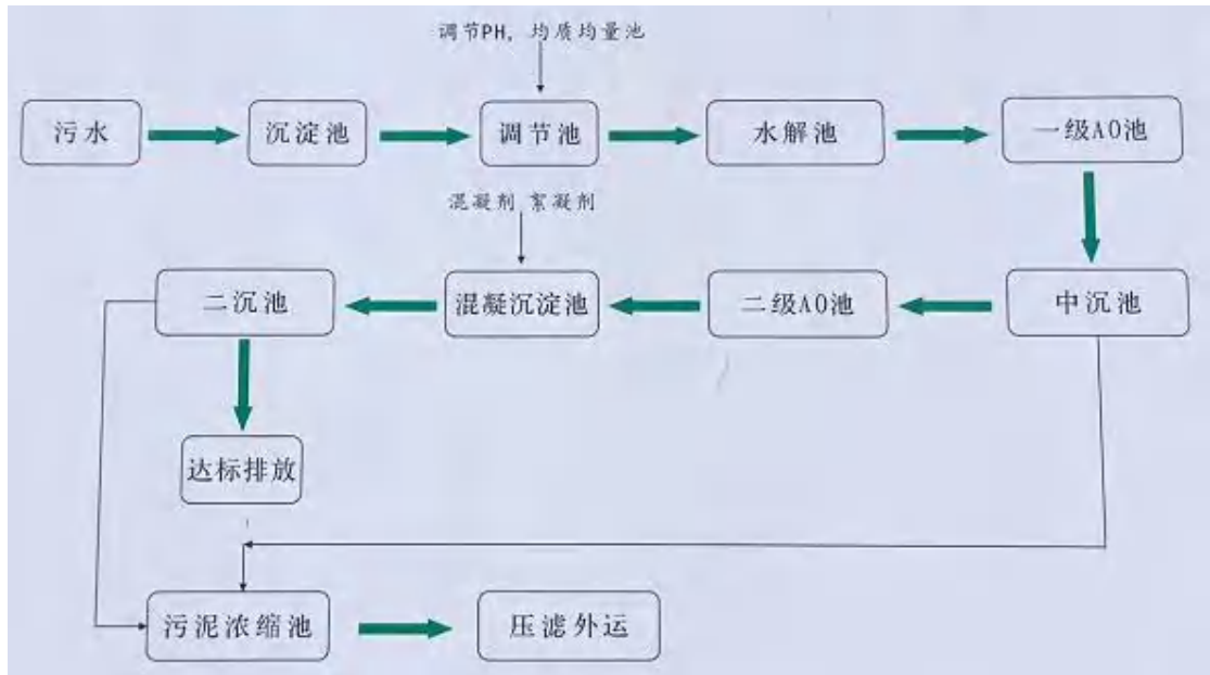
图 4.1-27 生产废水处理工艺图
