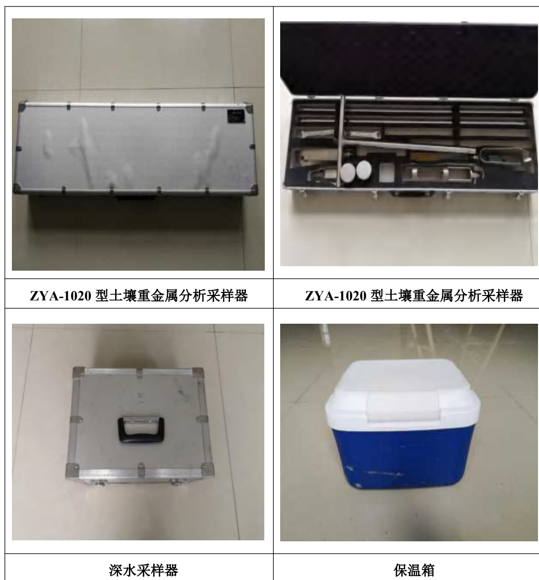
图 7.2-1 采样器具
