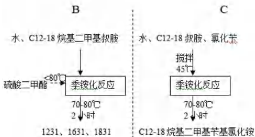
图 4.1-5 单链季铵盐系列阳离子表面活性剂生产工艺流程及产污位置图 双链季铵盐系列阳离子表面活性剂
