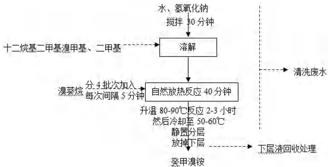
图 4.1-6 双链季铵盐系列阳离子表面活性剂生产工艺流程及产污位置图 苯扎溴铵
