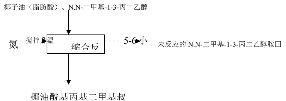
图 4.1-11 椰油酰基丙基二甲基叔胺生产工艺流程及产污位置图
